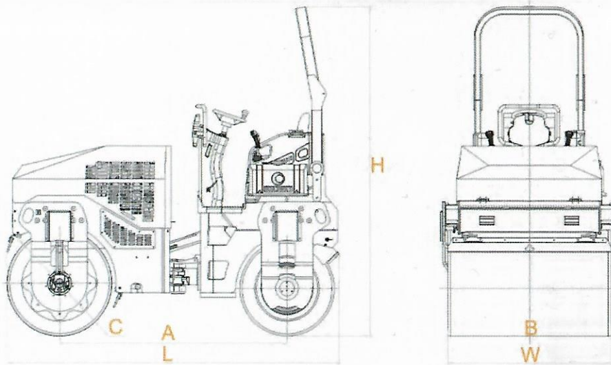
SRD04 / SRK04
